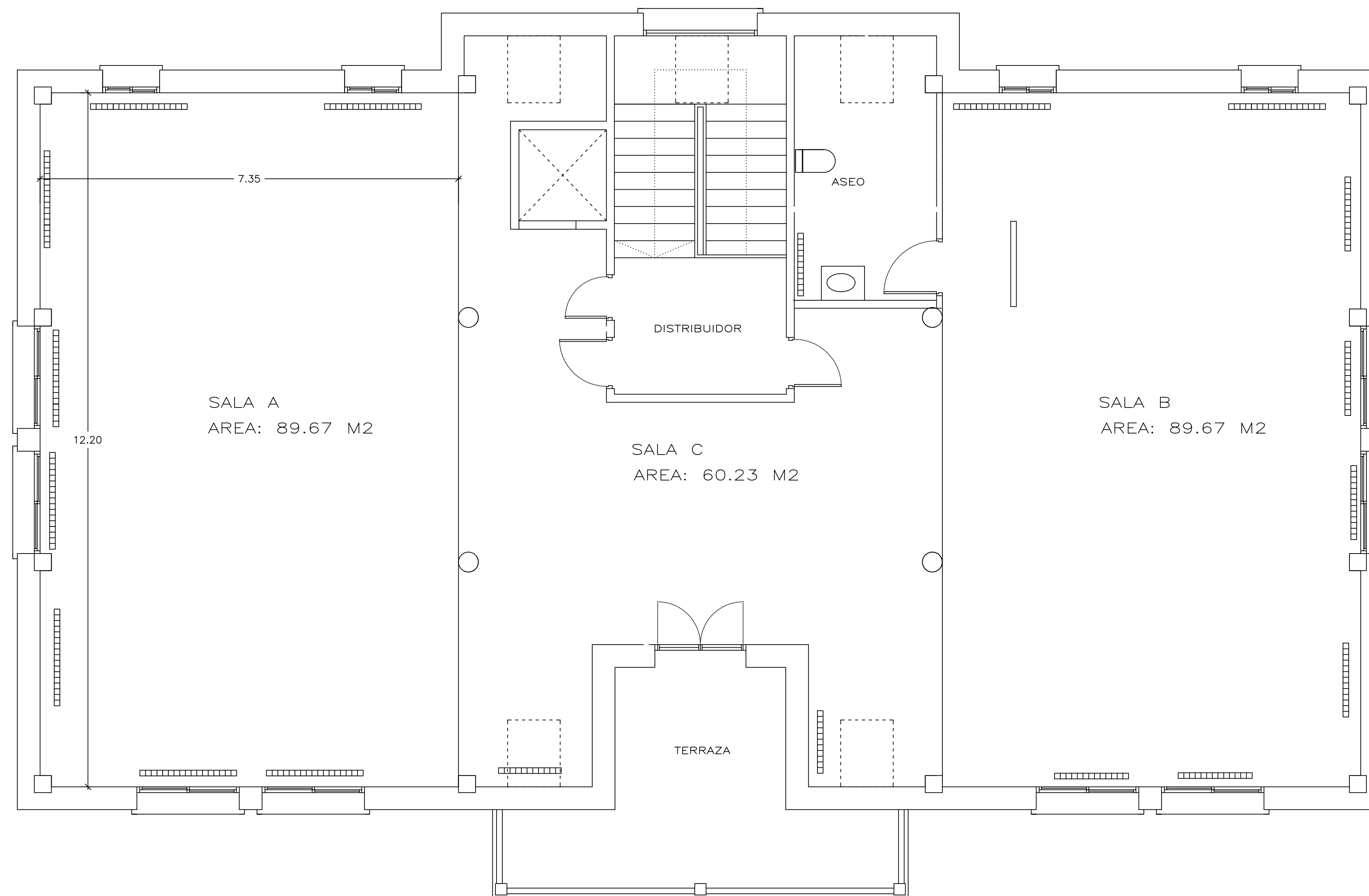
DISTRIBUCION PLANTA BAJO CUBIERTA
